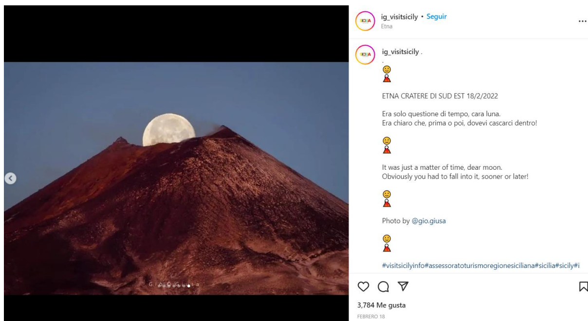
Slika 3: Vulkan Etna
